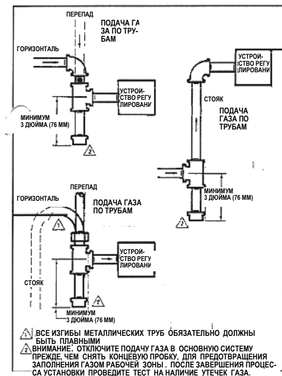
РИС. 4 – УСТАНОВКА ОТСТОЙНИКА
